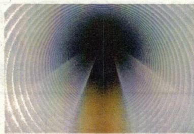
内側に帯状のプラスチックを巻き立て修理した下水道管
